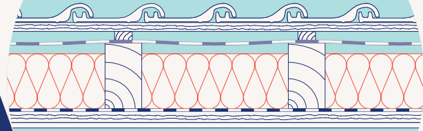
Belüftetes Dach (mit Hinterlüftung)
